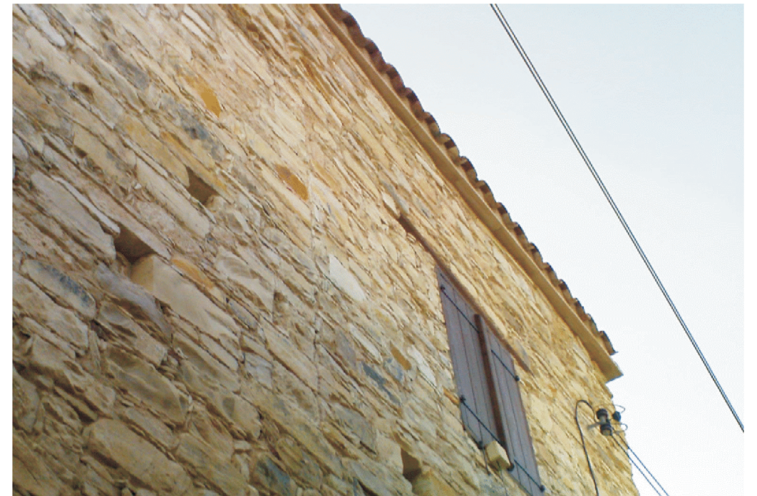
κρόδωμα κατασκευασμένο με προεξοχή των βολιτζιών από τη τοιχοποιία (με μεταγενέστερες επεμβάσεις)
